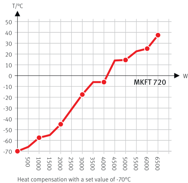
Wärmekompensationsdiagramm
